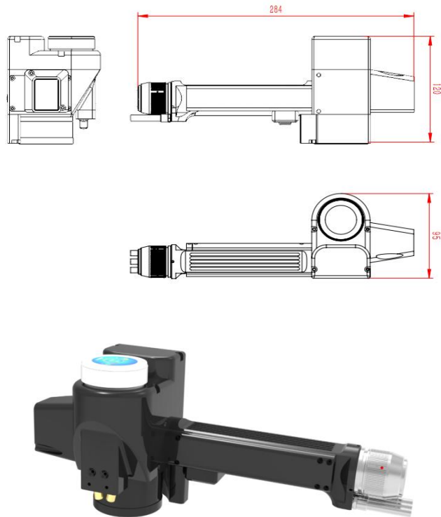
图 2 SKYCL-1-H-1000W 清洗头
