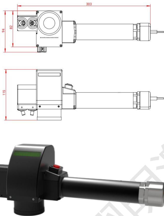
图 2 SKYCL-2-H-100A/200A/300A 清洗头
