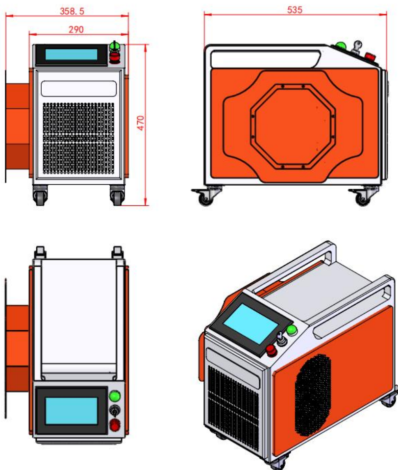
图 1 SKYCL-2-H-100A/200A/300A 外观图（产品以实际交付为准）
