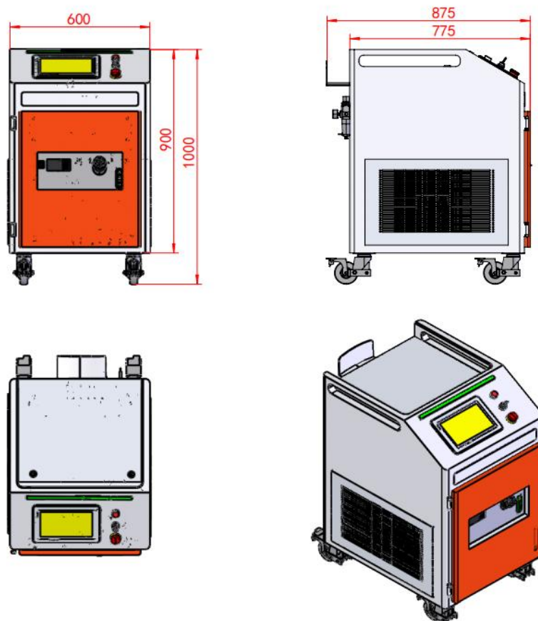
图1 SKYCL-1-H-500W 外观图（产品以实际交付为准）
