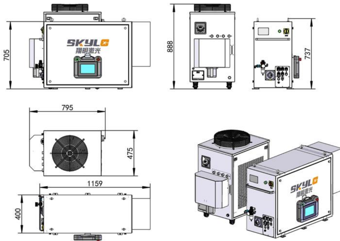
图 2 SKYLC-SPM-500/1000 分体式外观图（产品以实际交付为准）
