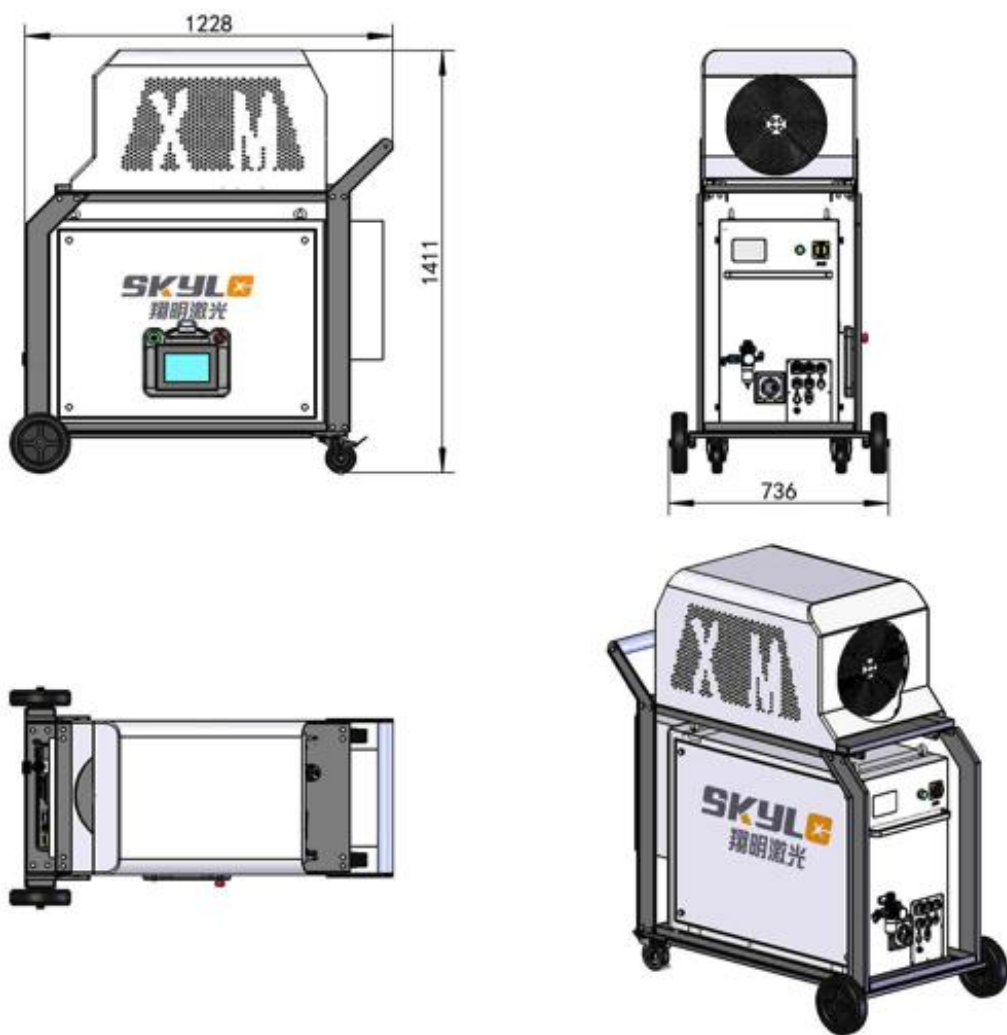
图1 SKYLC-SPM-2000 一体式外观图（产品以实际交付为准）
