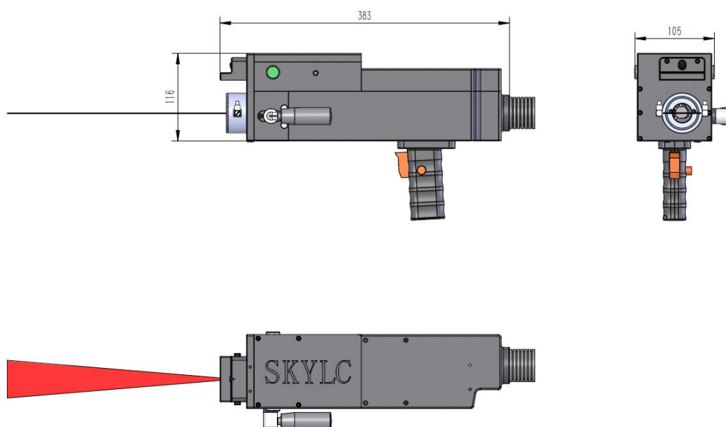
图 3 SKYLC-SPM-2000 清洗头
