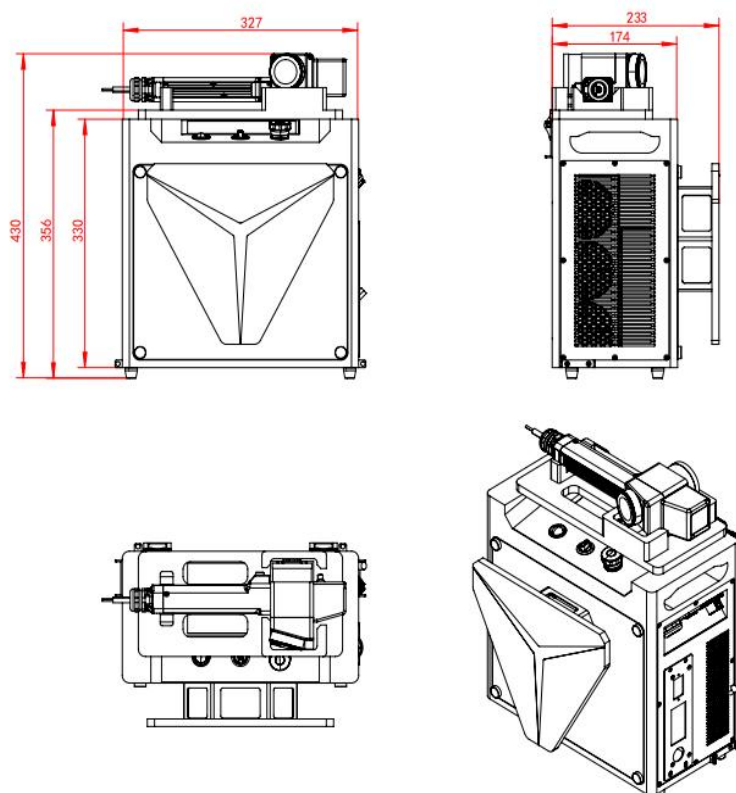
图 1 设备外观图（产品以实际交付为准）
