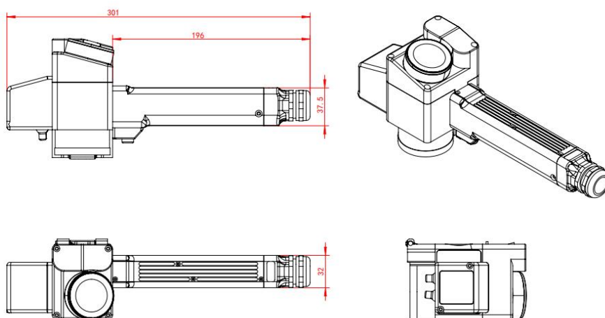
图1 设备外观图（产品以实际交付为准）
